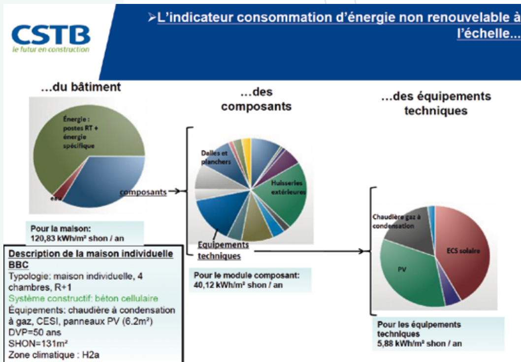
Figure 23 - Exemple de calcul des répartitions des consommations d'énergie non renouvelable – CSTB, Division Environnement – Assises nationales de l'énergie grise, 15 avril 2011
