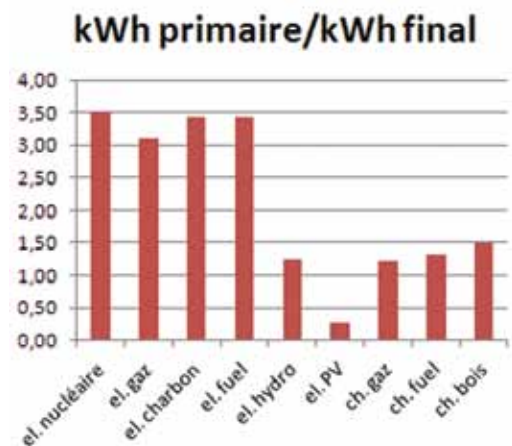
Figure 64 - Équivalences en énergie primaire par kWh final pour différentes énergies – Source : Bruno Peuportier, Centre Énergétique et Procédés, MINES ParisTech
