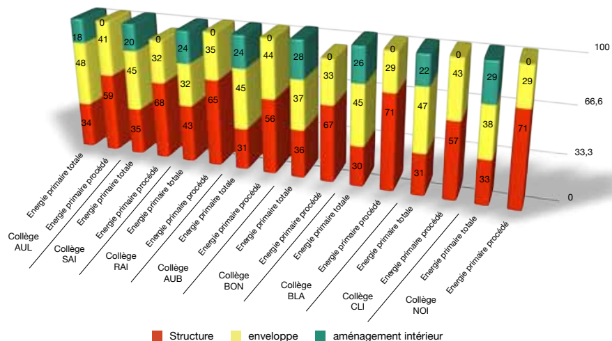
Figure 17 - Répartition des énergies par lot en pourcentage - Le Sommer Environnement
