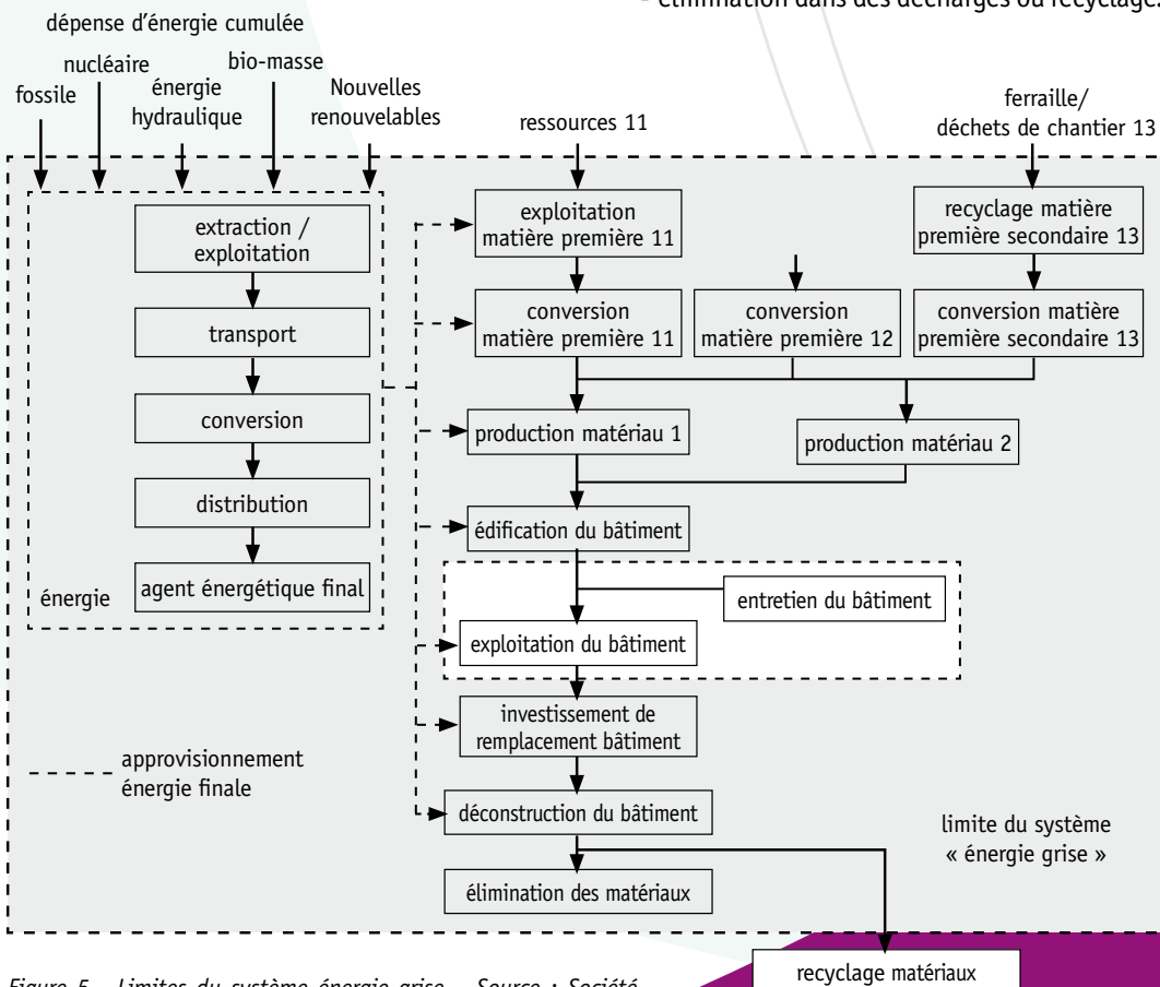
Figure 5 - Limites du système énergie grise – Source : Société des Ingénieurs et Architectes, SIA - Cahier Technique, CT 2032 – 2010
