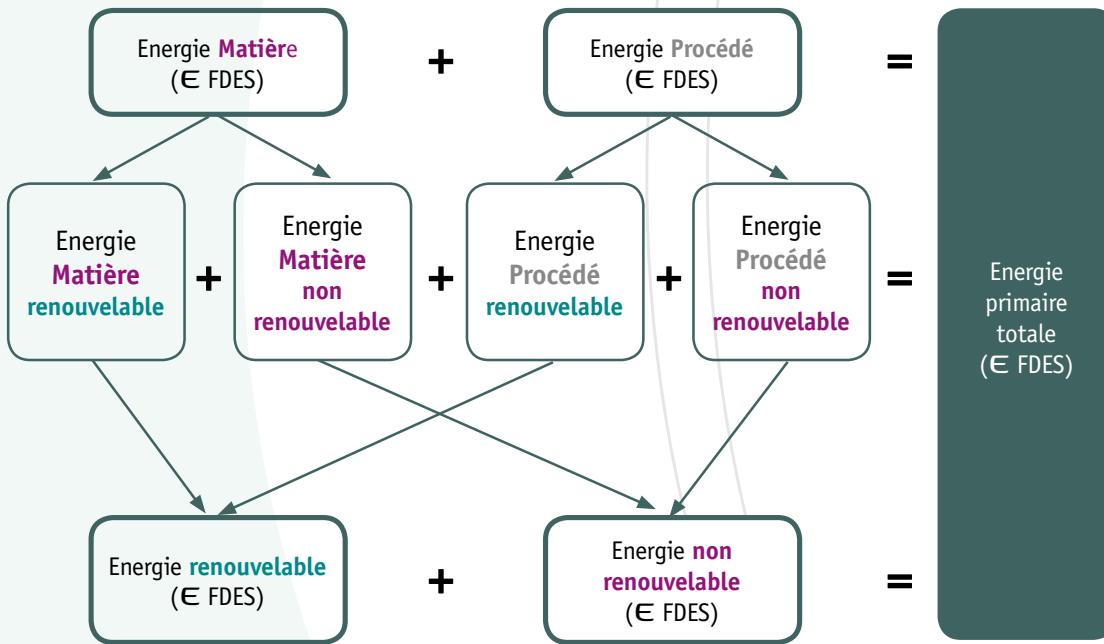
Figure 6 - Les différentes énergies qui composent l'énergie grise - FCBA, Claire Corniller - ICEB Café du 27/10/2009
