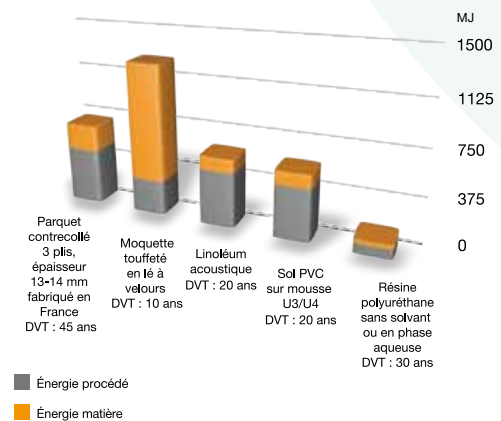
Figure 9 - Comparaisons entre énergies primaire totale, énergie procédé et énergie matière pour des revêtements de sol - AILTER, 2011
