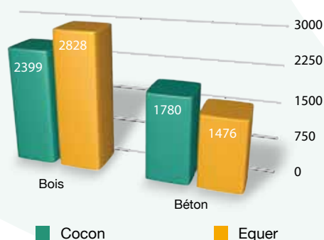
Figure 43 – Étude comparative de deux variantes structurelles pour le bâtiment du CE à Roissy avec les logiciels ELODIE et Cocon – Graphique ICEB à partir des données du rapport d'H. Leh
