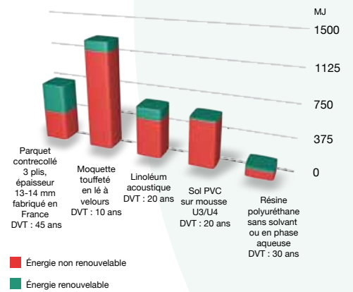
Figure 8 - Comparaisons entre énergies primaire totale, énergie renouvelable et non renouvelable pour des revêtements de sol - AILTER, 2011
