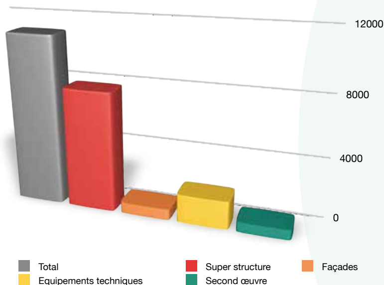
Figure 20 - Construction d'un bâtiment à usage mixte (commerces, bureaux et logements – Calcul des émissions de GES pour la construction - SYMOE
