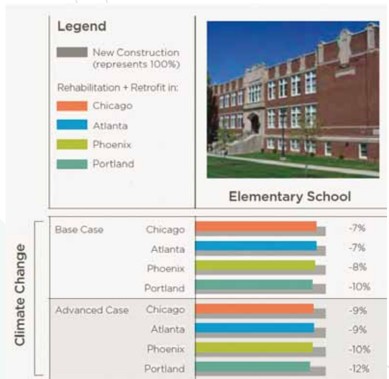
Figure 26 - the greenest building : émissions de gaz à effet de serre comparées entre réhabilitation et construction neuve pour des écoles
