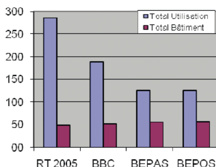
Figure 31 - Comparaison en énergie primaire totale (kWh/m 2 .an) sur une durée de vie de 30 ans du même bâtiment, SSLIA de Roissy avec des performances énergétiques différentes - Source : Évaluation des Impacts Environnementaux des Bâtiments Au niveau Structure et Matériaux – Rapport de stage Hélène Leh - ADP / INP ENSEEIHT – Septembre 2010
