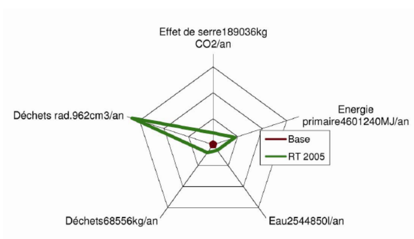
Figure 30 – Impacts comparés du projet à énergie positive (base) et de la même opération respectant uniquement la RT 2005 - Ville de Pantin – Construction de l'école du centre – Simulation de l'impact environnemental – MÉANDRE – Juillet 2008
