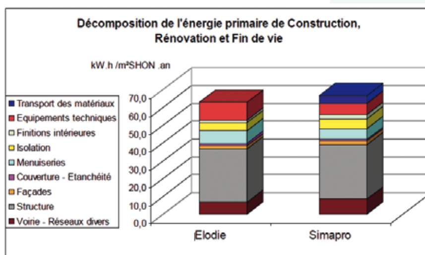
Figure 44 - Étude COIMBA - Décomposition de l'énergie primaire pour la maison des Hauts de Feuilley - Comparaison des résultats obtenus avec ELODIE et SIMAPRO
