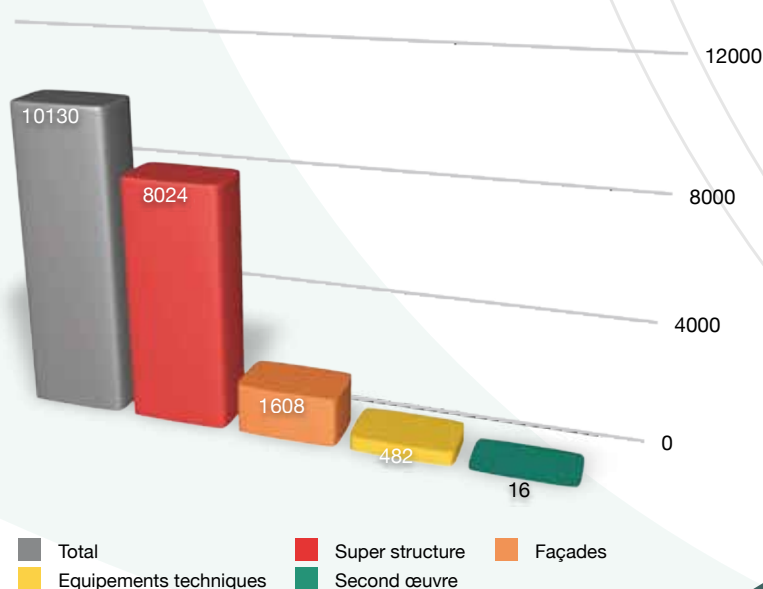
Figure 18 - Projet de réhabilitation d'entrepôts en bureaux – Calcul des émissions de GES pour la réhabilitation/reconversion - SYMOE
