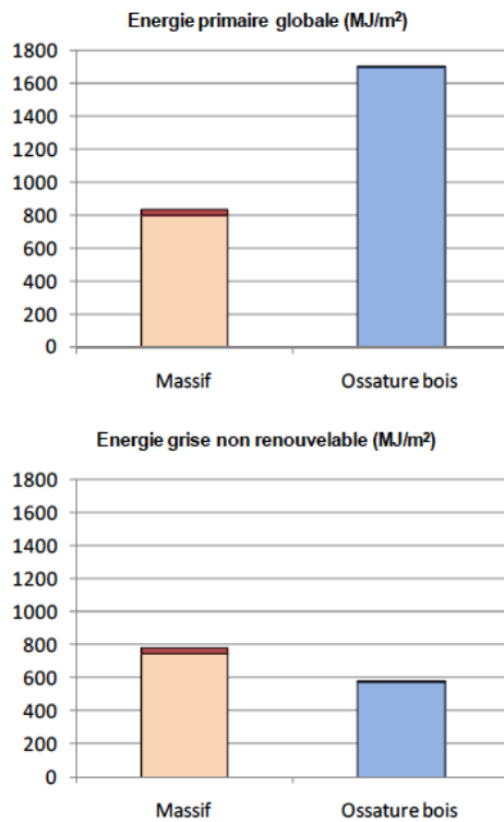
Figure 7 - Comparaison de l'énergie grise de deux parois verticales – L'énergie grise des bâtiments – Weinmann-Energies SA, Francine Gass – Lunch-débat – 18 juin 2010
