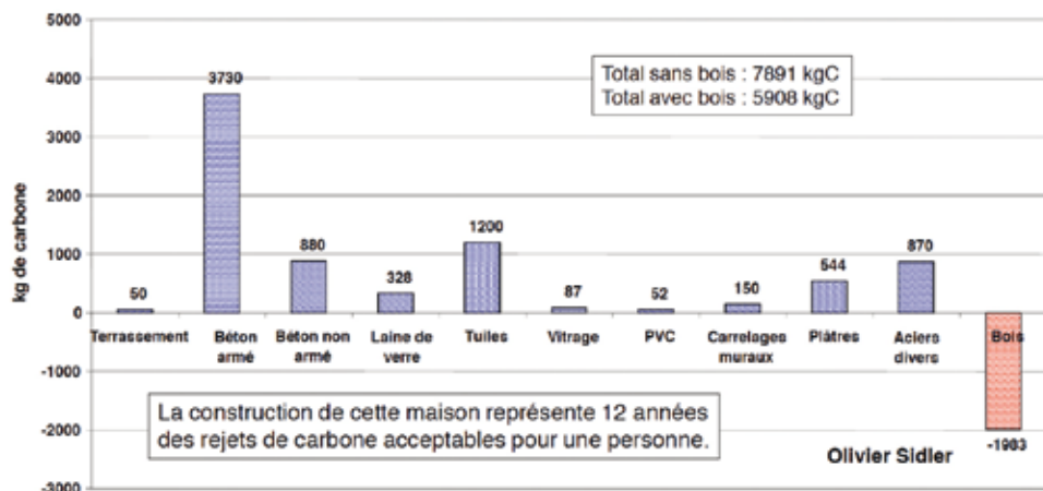
Figure 25 – Les émissions de gaz à effet de serre en équivalent carbone liées à la construction d'une maison individuelle – ENERTECH
