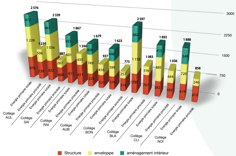
Figure 16 - Répartition des énergies par famille (en kWh/m 2 SHON) - Le Sommer Environnement
