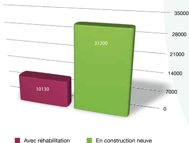
Figure 19 - Comparaison des émissions de GES entre réhabilitation et construction neuve pour des bureaux - SYMOE
