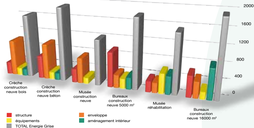
Figure 15 - Calculs TRIBU : bilan des consommations en énergie grise, totale et poste par poste, en kWh/m 2 shon sur 50 ans de durée de vie du bâtiment
