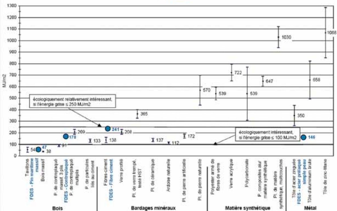
Figure 32 - Énergie grise des bardages - Source : éco-devis 343 édité par l'association de soutien eco-devis - juin 2008 complété par AILTER avec des valeurs issues des FDES
