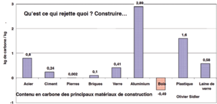
Figure 53 - Impact carbone de matériaux de construction - Source : ENERTECH
