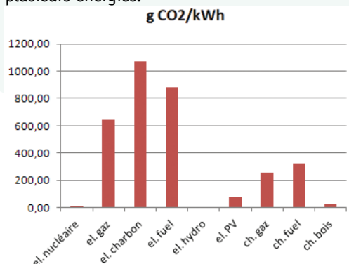
Figure 2 : Émissions de gaz à effet de serre en équivalent CO 2 par kWh d'énergie finale pour différentes énergies – Source : Bruno Peuportier, Centre Énergétique et Procédés, MINES ParisTech
