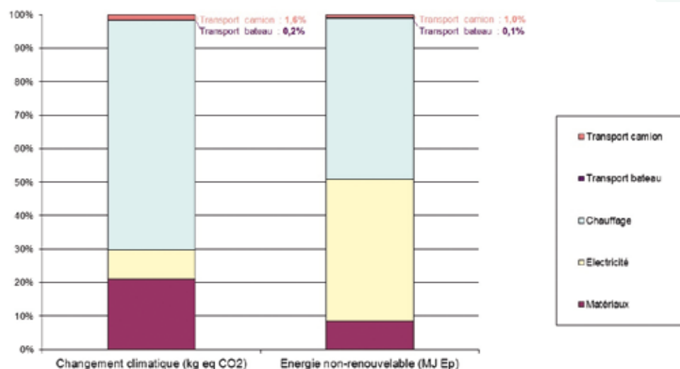
Figure 22 - Étude COIMBA : impact des différentes phases du cycle de vie sur l'énergie primaire non renouvelable pour une maison individuelle conforme à la RT 2005
