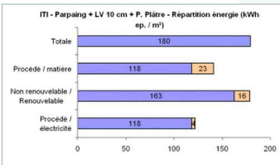
Figure 50 : COCON - Contenu en énergie grise d'une paroi en parpaings isolés par l'intérieur. Source : http://www.eosphere.fr/COCON-Les-onglets-de-description.html
