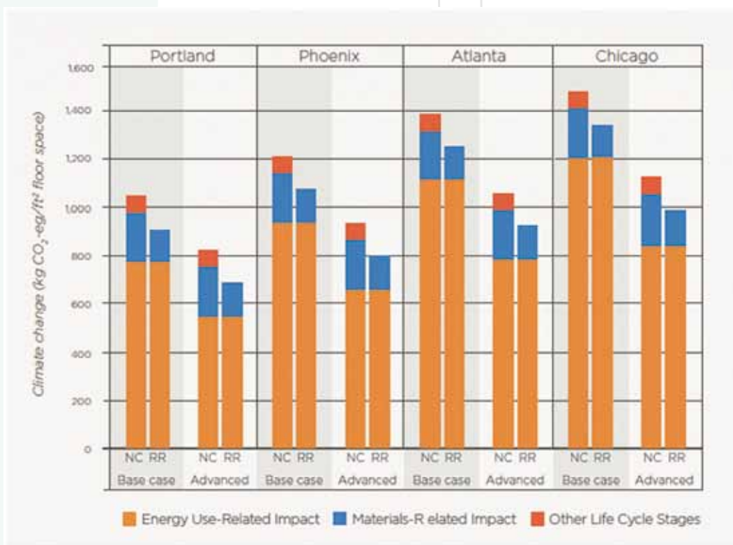
Figure 28 – The greenest building – Comparaison des émissions de gaz à effet de serre globales entre un bâtiment à performance énergétique standard et un bâtiment 30 % plus performant pour la construction neuve (NC) et la réhabilitation (RR)
