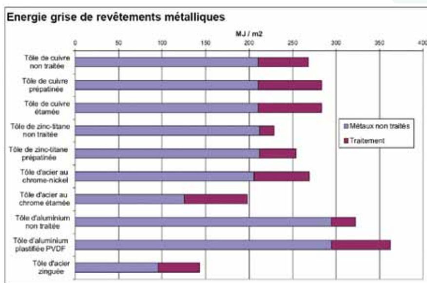
Figure 55 - Énergie grise des revêtements métalliques - Source : éco-devis 343 édité par l'association de soutien éco-devis - juin 2008
