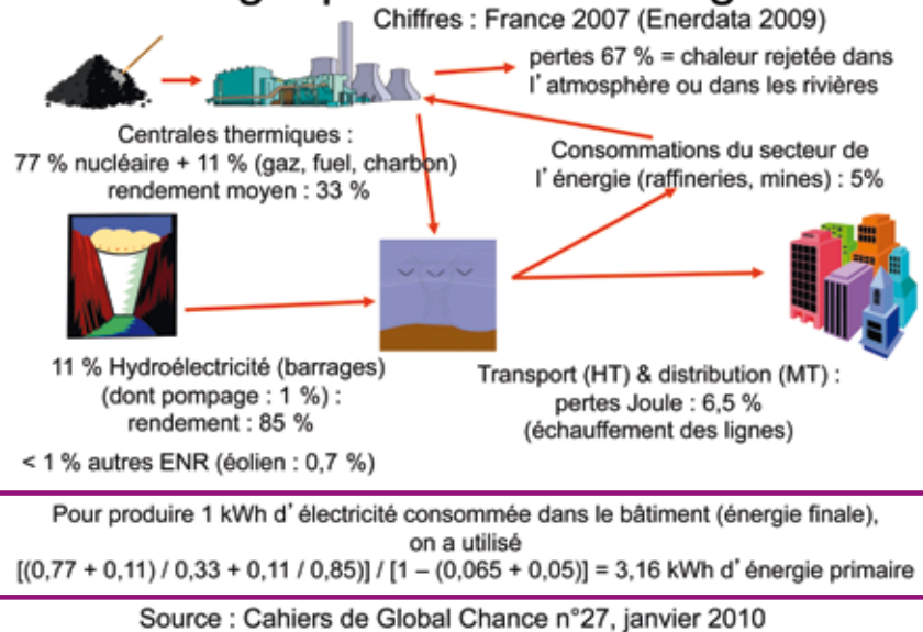
Figure 63 - Calcul du Facteur d'Énergie Primaire (PEF) du mix électrique français (Sidoroff, 2012)
